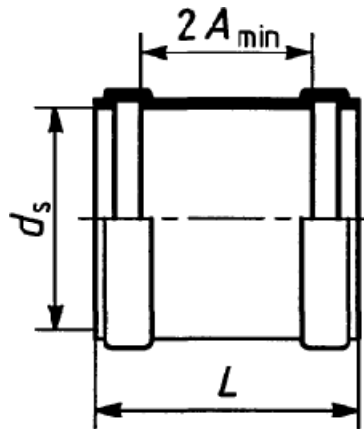
شکل ۱۳- جفت ساز لغزشی
