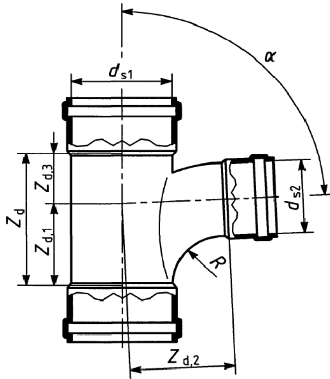
شکل ۱۷- انشعاب‌گیر تمام مادگی کاهنده (بدون ناحیه مرده)
