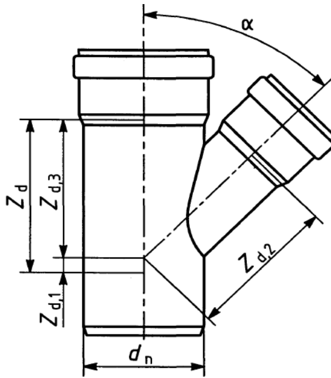
شکل ۱۸- انشعاب‌گیر کاهنده (دارای ناحیه مرده)
