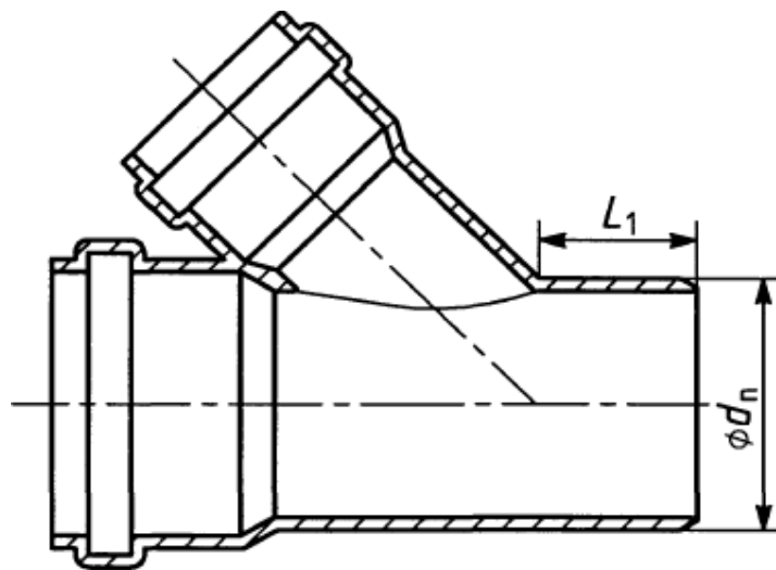
شکل ۵- طول های نری
