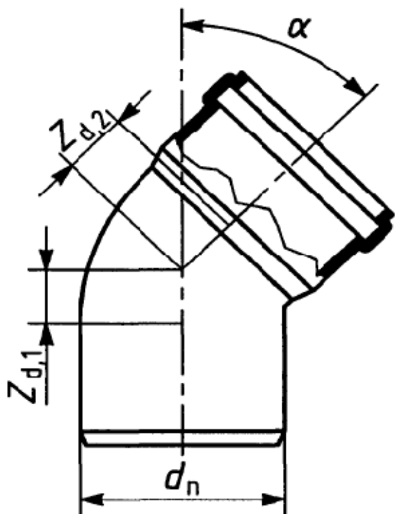
شکل ۷- خم با یک مادگی (دارای ناحیه مرده)
