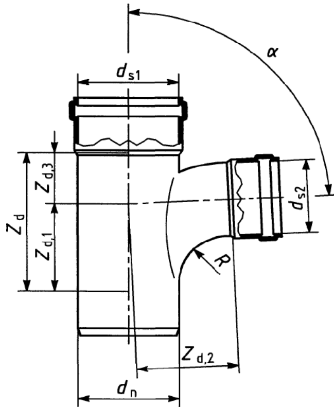
شکل ۱۶- انشعاب‌گیر کاهنده (بدون ناحیه مرده)
