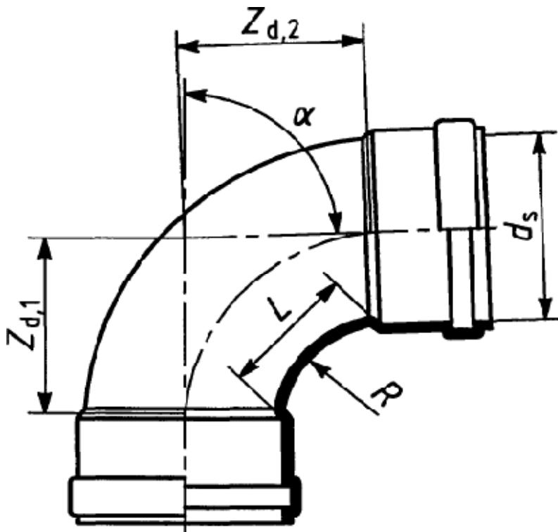
شکل ۹- خم تمام مادگی (بدون ناحیه مرده)
