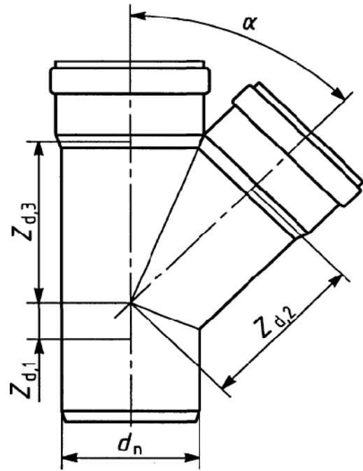
شکل ۱۵- انشعاب‌گیر (دارای ناحیه مرده)
